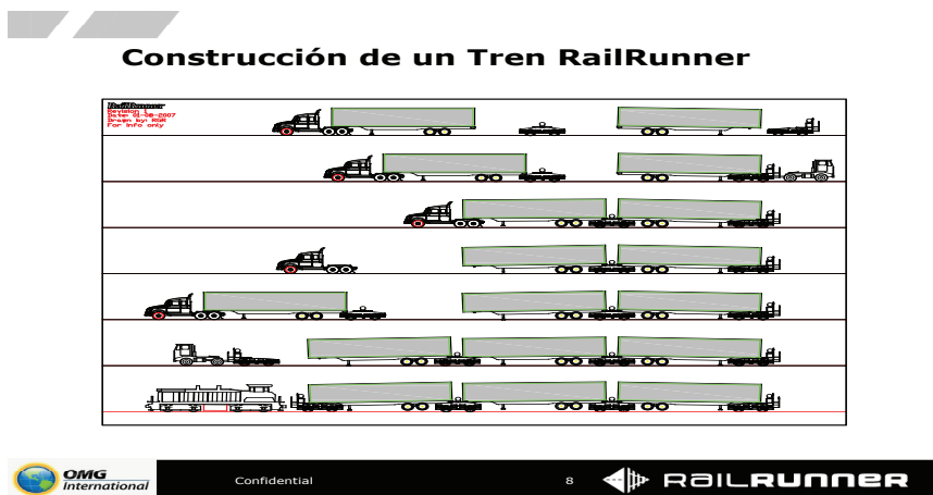
Figura 4 Construcción de un tren rail runner
